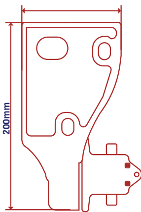
VISTA TRASERA 101mm
