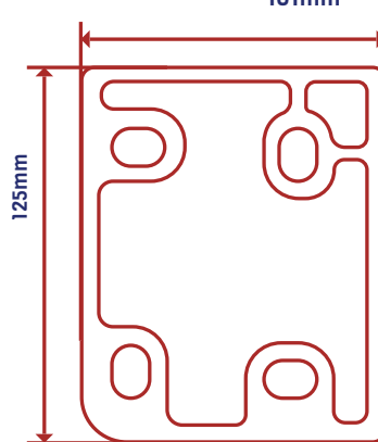
VISTA SUPERIOR 101mm
